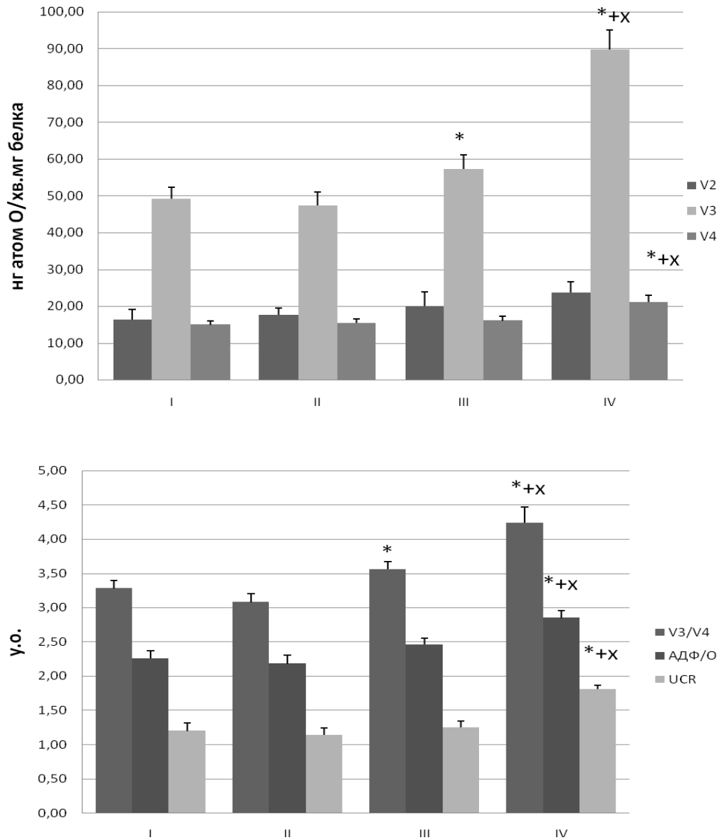
Рисунок 5.4. Зміни показників дихання мітохондрій при окисненні Гм у щурів I-IV груп. * P < 0.05 в порівнянні з I групою, ^x P < 0.05 в порівнянні з II групою, ^+ P < 0.05 в порівнянні з III групою.
