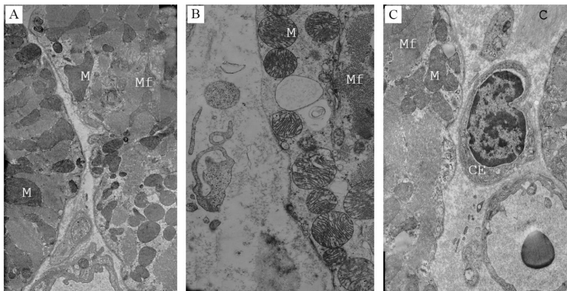
Рис.6.7 Ультраструктура міокарду лівого шлуночка серця щурів групи SHR. Дезорганізація мітохондрій, які в значній мірі відрізняються за розмірами та ступенем пошкодження, в розширеному, заповненому колагеном міжклітинному просторі залишки клітин із цілісною цитоплазматичною мембраною невизначеного походження. А - зб.Х5000; В - зб.Х7200; С - зб.Х5000. Мf- міофіламенти, М-мітохондрії, СЕ - ендотелій капіляру.
