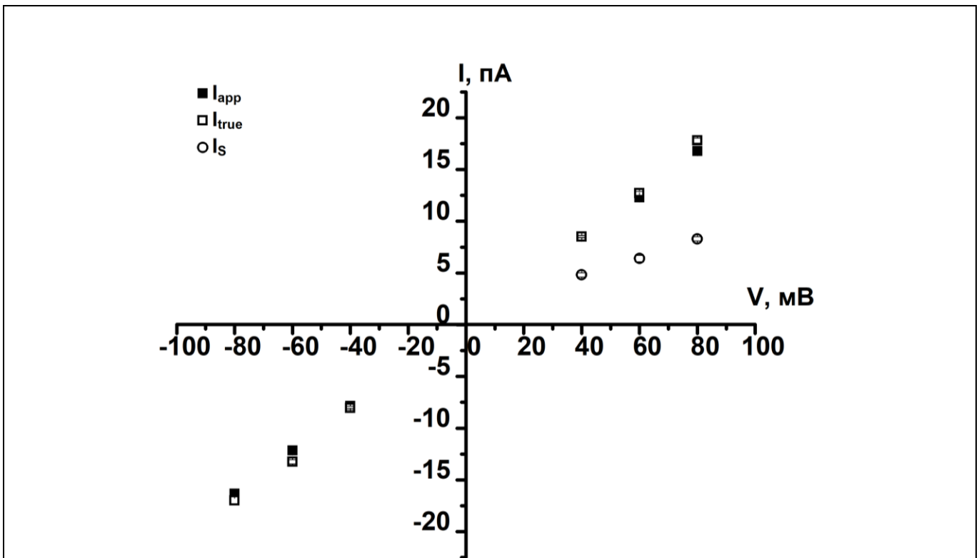
Рис. 3.31. Вольт-амперна характеристика LCC-каналів. Чорним кольором на графіку показано видиму амплітуду струму, визначену як різницю амплітуди струму між рівнями провідності іонного каналу за допомогою курсорів у Clampfit. Справжню амплітуду було визначено в результаті аналізу \beta -розподілу ( n=4-5 ).
