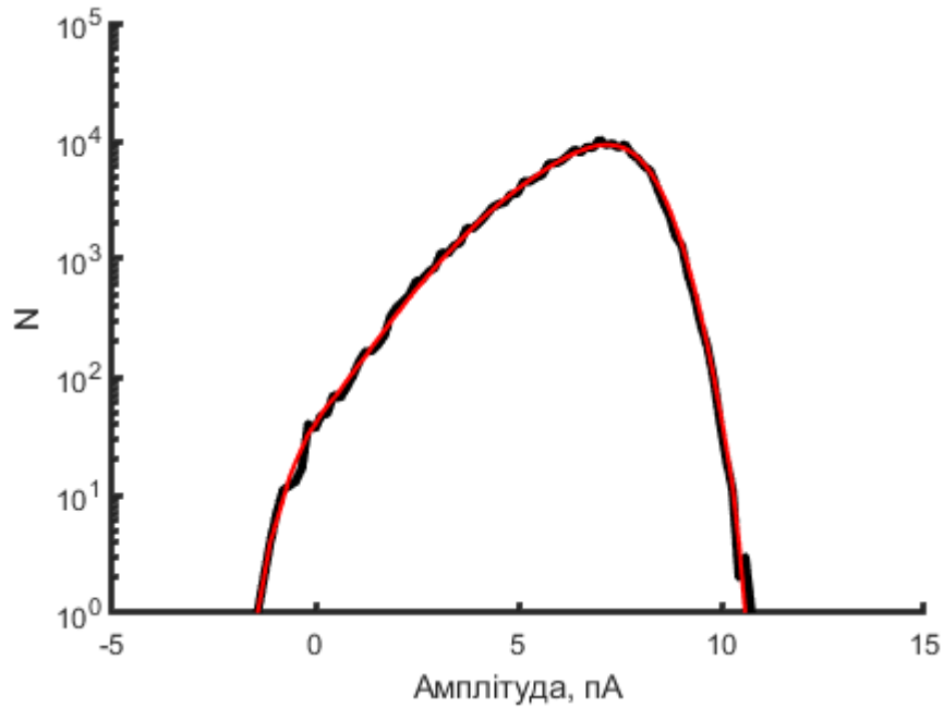
Рис. 3.33. Накладання теоретичної кривої амплітудної гистограми на експериментальну в результаті аналізу \beta -розподілу при дії концентрації 1 мМ галламіну при мембранному потенціалі +40 мВ. Швидке блокування галламіном викликає сильне зменшення амплітуди струму внаслідок збільшення шуму відкритого стану. Теоретична крива (червоного кольору) була підібрана з константами асоціації k_{on}=10623 \text{ c}^{-1} та дисоціації k_{off}=51943 \text{ c}^{-1} .
