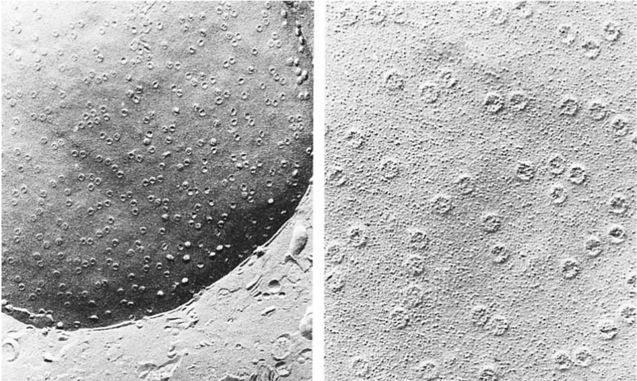
Рис. 1.2. Мікрофотографія, зроблена з використанням низьковольтного електронного мікроскопа, що показує типовий вигляд ядра клітини Пуркіньє (внутрішньої мембрани) з ядерними порами; зліва збільшення \times 17000 , справа ділянка із збільшенням \times 56000 (За [84])
