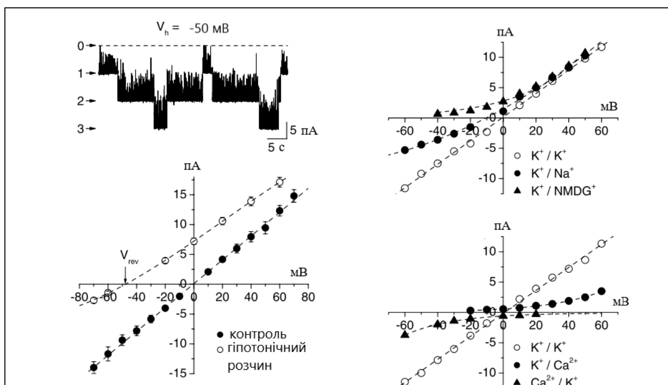
Рис. 1.3. Властивості LCC-каналів на ядерній оболонці нейронів Пуркінє мозочка щура. Потенціал реверсії LCC-каналів складає -48,6 \text{ мВ} в гіпотонічному розчині. Канали селективні до одновалентних катіонів та непроникні для двовалентних катіонів та великих молекул як \text{MNDG} (За [20]).
