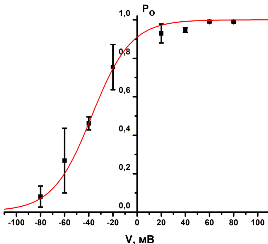
Рис. 3.23. Ймовірність відкритого стану ( P_o ) LCC-каналів за умови наявності лише одного каналу в петчі. Експериментальні точки були отримані за стаціонарних умов при потенціалах -80\text{ мВ} ( n=6 ), -60\text{ мВ} ( n=3 ), -40\text{ мВ} ( n=22 ), -20\text{ мВ} ( n=8 ), +20\text{ мВ} ( n=9 ), +40\text{ мВ} ( n=31 ), +60\text{ мВ} ( n=7 ), +80\text{ мВ} ( n=4 ).
