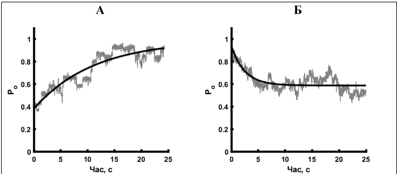
Рис. 3.22. Час затримки перед першим закриванням та відкриванням LCC-каналів (латентність) при зміні потенціалу з -80 мВ на +80 мВ (А) та +80 мВ на -80 мВ (Б). Для визначення \tau було використано петчі з одним каналом n=11 для переходу до +80 мВ та n=4 для переходу до -80 мВ.
