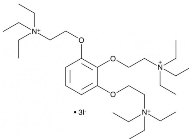
Рис. 3.13. Структурна формула галламіну триетіюідиду.
