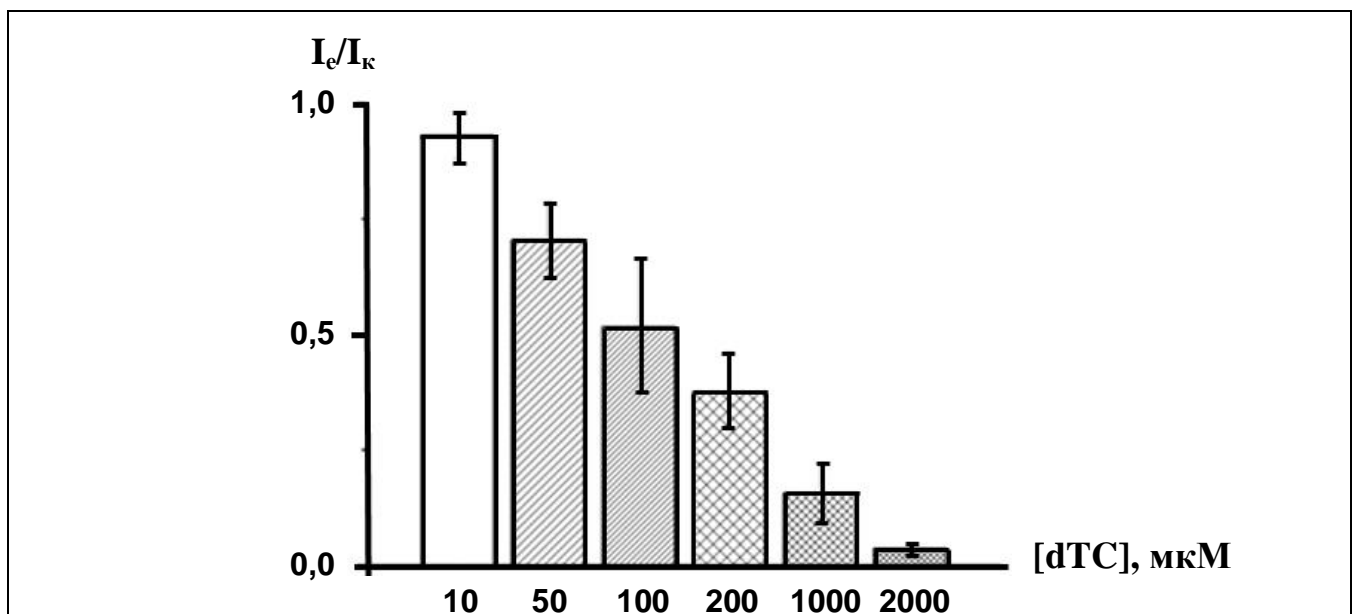
Рис. 3.12. Вплив dTC на LCC-канали. Співвідношення видимої амплітуди струму в контролі та у за умови дії різних концентрацій dTC в діапазоні від 10 мкМ до 2 мМ при фіксованому потенціалі -40 мВ (n=4-5).
